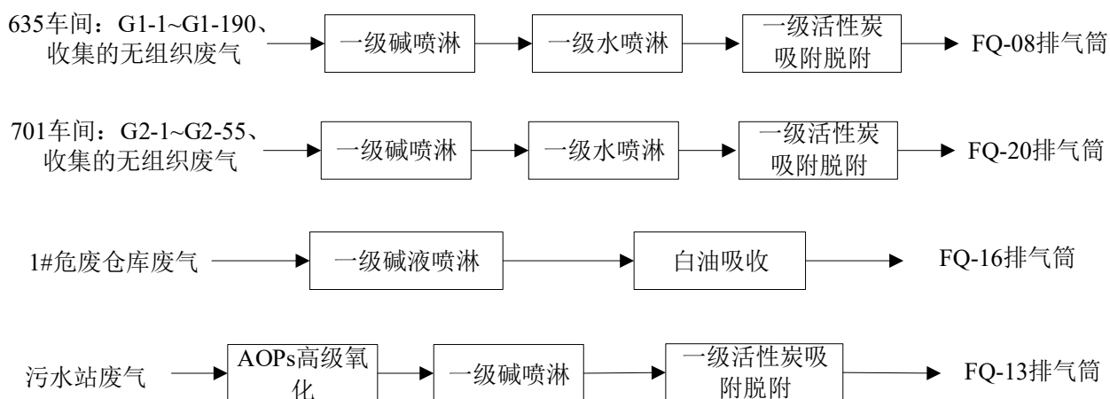
图 7.2-1 项目车间有组织废气污染物走向情况
